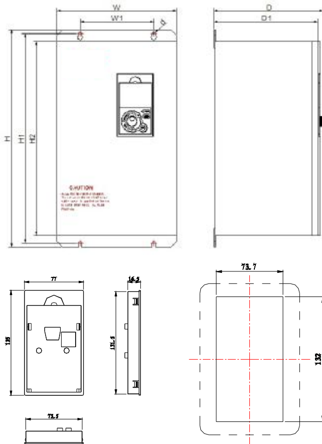
图 2-1 AMB500F 外形尺寸和安装尺
