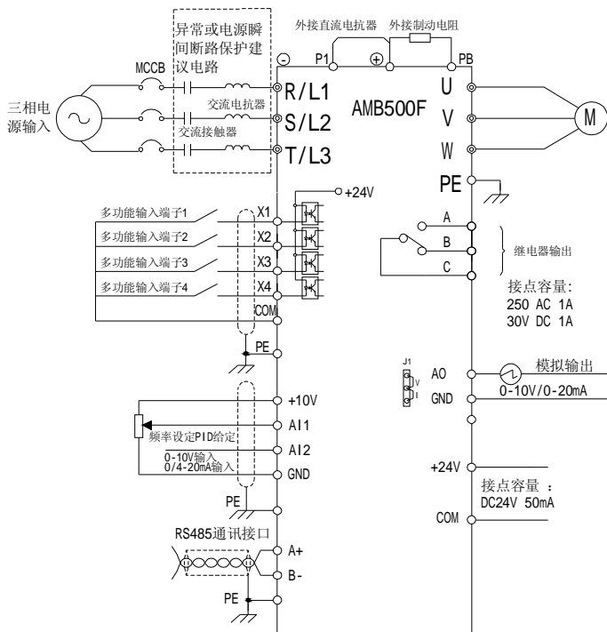
图 3-2-2 AMB500F (11-132KW) 变频器连接图
