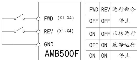
图 7- 3 2 线制顺序控制 1
