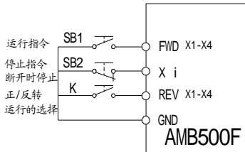
图 7- 6 3 线制顺序控制模式 2
