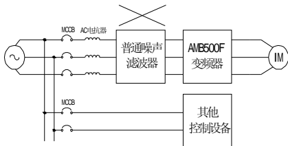
图 3-5 噪声滤波器的正确设置
