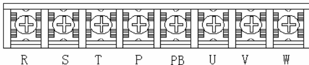
三相 220V/380V(0.75-7.5KW)主回路端子
