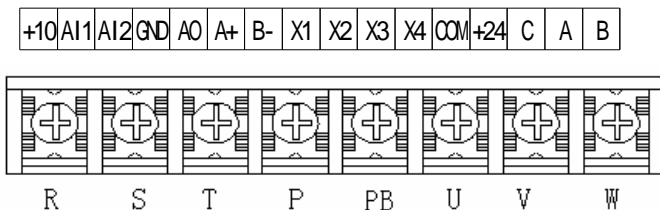
三相 220V/380V(0.75-7.5KW)主回路端子 图 1-2 控制回路端子和主回路端子配置
