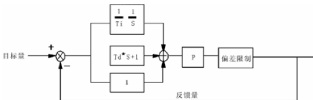
图 7-18 过程 PID 原理框图
