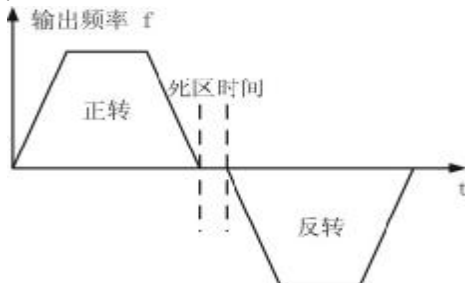
图 7-10 正反转死区时间示意图
