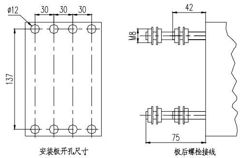
HM3-160R 板后接线
