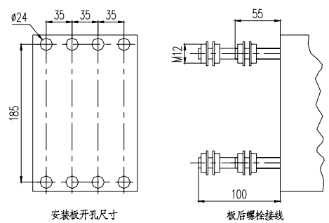
HM3-250R 板后接线
