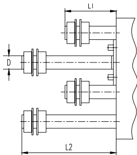
板后螺杆式接线俯视图
