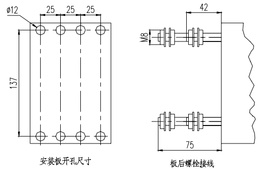
HM3-100R 板后接线
