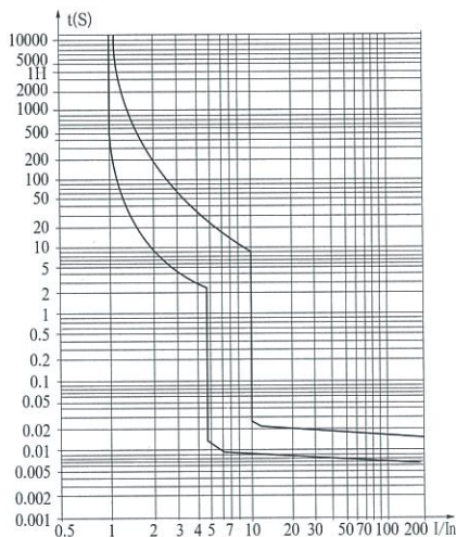
HB45L-32N型曲线(5 ~ 10In)
