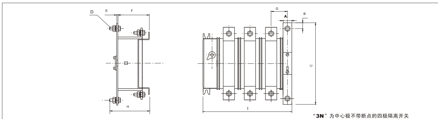
“3N”为中心极不带断点的四极隔离开关
