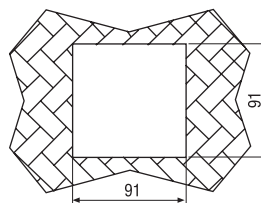
面板开孔尺寸
