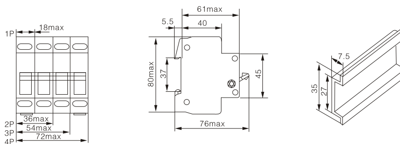
图1 CFH2-125 小型隔离开关外形及安装尺寸
