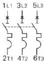
图 3 断路器主接线图
