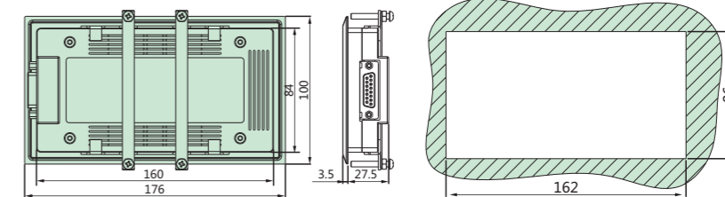
控制器分体部分外形尺寸
