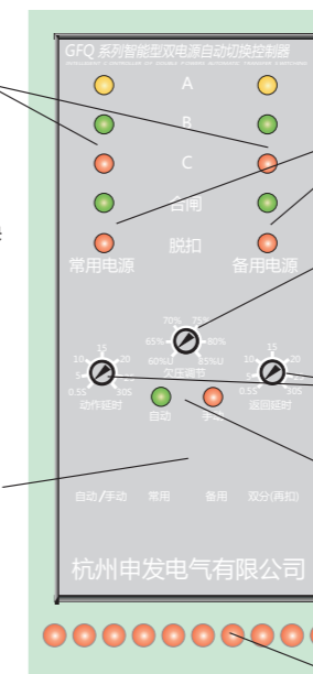
Y型控制器
