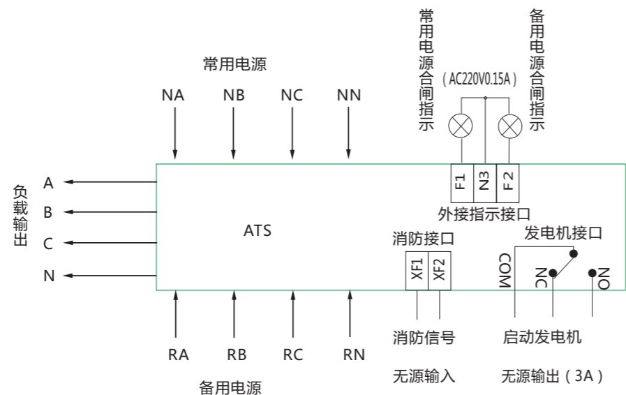
GFQ1-63Y用户接线示意图
