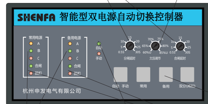
F型控制器
